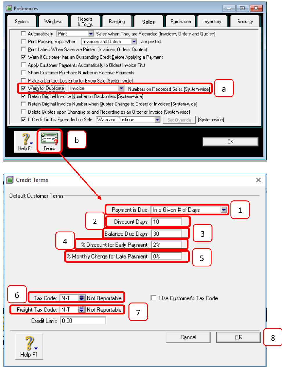
Gambar 3.6. Tampilan Preferensi Sales
