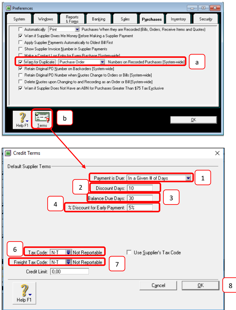
Gambar 3.7. Tampilan Preferensi Purchases
