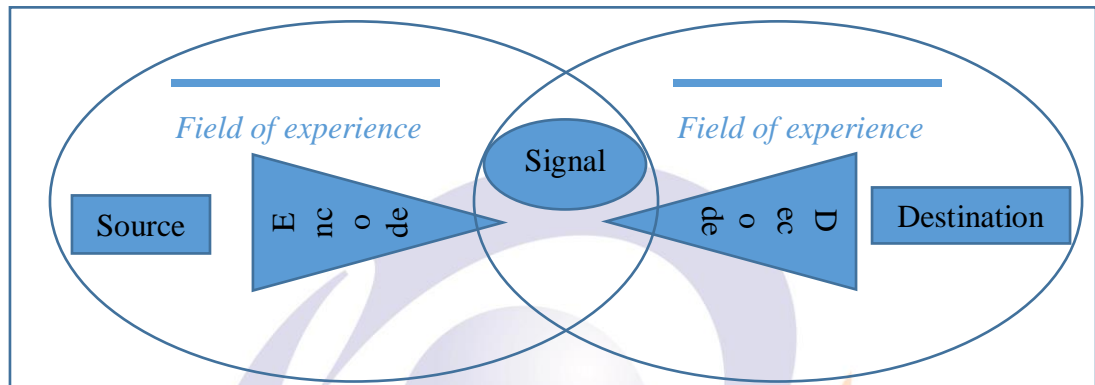
Gambar 2. Model Schramm
